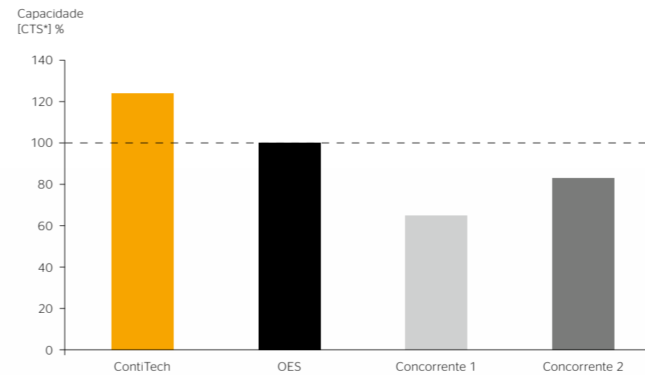
Comparação entre as bombas de água da ContiTech, da OES e da concorrência
